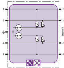
Prinzipschaltbild BXT ML4 MY 110
