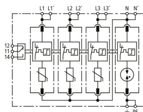
Prinzipschaltbild DG MD TT 275 FM
