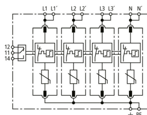
Prinzipschaltbild DG MD TNS 275 FM
