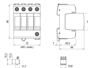
Maßbild DG MD TNS 275 FM
