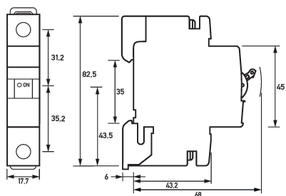
Maßzeichnung Leitungsschutzschalter DLS 6i Co,5-1
