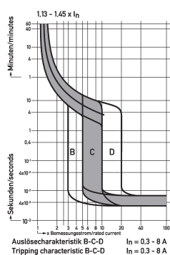
Diagramme Leitungsschutzschalter DLS 6i Co,5-1
