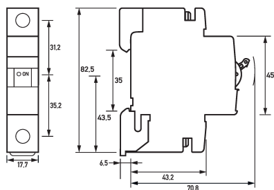
Maßzeichnung Leitungsschutzschalter DLS 6h B32-1
