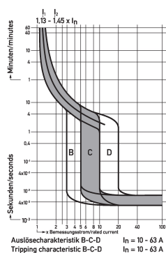
Diagramme Leitungsschutzschalter DLS 6h B32-1
