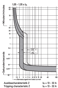
Diagramme Leitungsschutzschalter DLS 6i Z32-3
