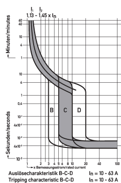
Diagramme Leitungsschutzschalter DLS 6h C10-3
