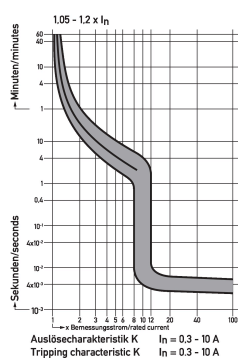
Diagramme Leitungsschutzschalter DLS 6i K2-2
