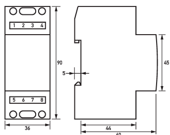
Maßzeichnung Klingeltransformatoren RK 24
