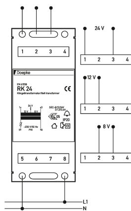
Schaltungsbeispiel Klingeltransformatoren RK 24
