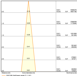
FL MAX P 1200W 740 R10 WAL
