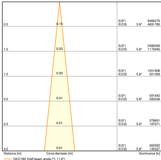
FL MAX P 900W 740 R10 WAL
