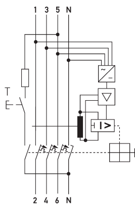
Schaltungsbeispiel FI-/LS-Kombinationen DRCBO 4 B16/0,03/3N-B NK
