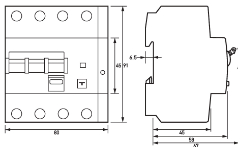
Maßzeichnung FI-/LS-Kombinationen DRCBO 4 B16/0,03/3N-B NK
