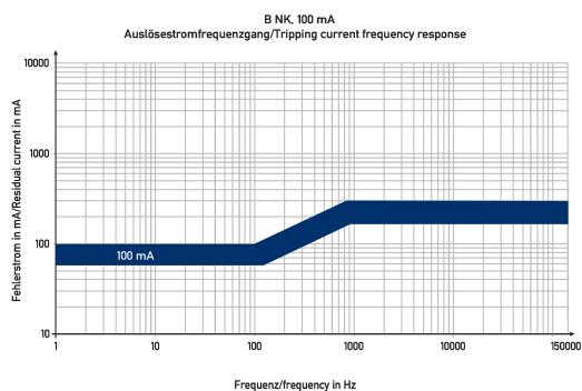
Diagramme FI-/LS-Kombinationen DRCBO 4 B10/0,10/1N-B NK
