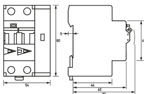
Maßzeichnung Fehlerlichtbogen-Schutzeinrichtungen DAFDD 1 B20/0,03/2-A
