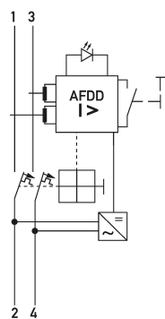
Schaltungsbeispiel Fehlerlichtbogen-Schutzeinrichtungen DAFDD 1 B20/0,03/2-A
