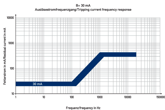
Diagramme FI-/LS-Kombinationen DRCBO 4 B16/0,03/3N-B+
