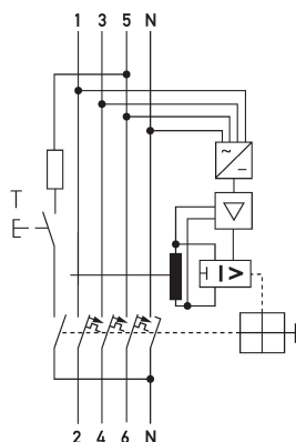
Schaltungsbeispiel FI-/LS-Kombinationen DRCBO 4 B16/0,03/3N-B+
