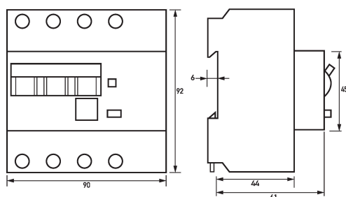
Maßzeichnung FI-/LS-Kombinationen DRCBO 4 B40/0,03/3N-A
