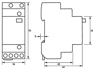
Maßzeichnung Installationsrelais RI 024-002
