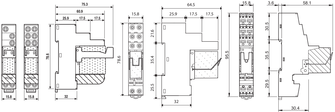
Typ 48.31 / 48.32 / 48.52 / 48.61 / 48.62 Schraubklemmen
