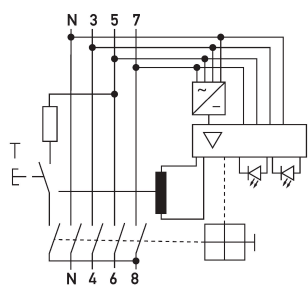
Schaltungsbeispiel Fehlerstromschutzschalter DFS 6 040-4/0,03-A NU
