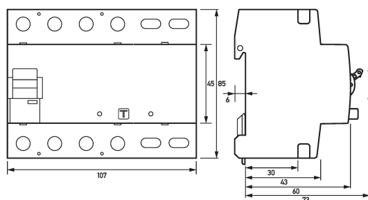
Maßzeichnung Fehlerstromschutzschalter DFS 6 040-4/0,03-A NU
