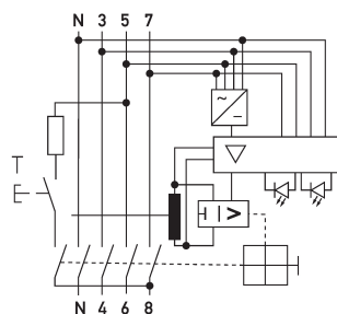
Schaltungsbeispiel Fehlerstromschutzschalter DFS 6 040-4/0,03-B SK NU
