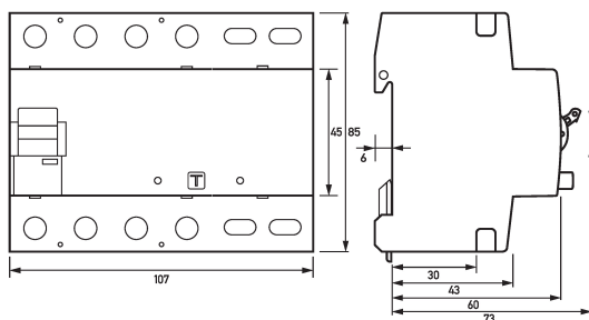
Maßzeichnung Fehlerstromschutzschalter DFS 6 040-4/0,03-B SK NU
