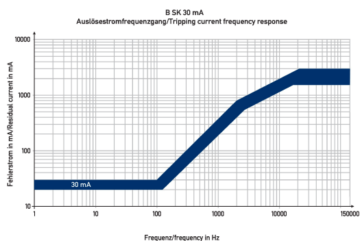
Diagramme Fehlerstromschutzschalter DFS 6 040-4/0,03-B SK NU
