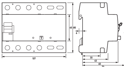
Maßzeichnung Fehlerstromschutzschalter DFS 6 063-4/0,03-B SK NU
