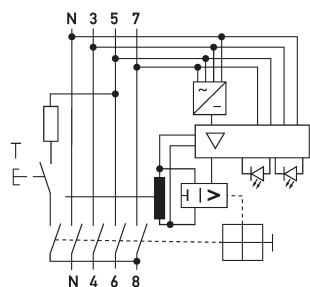
Schaltungsbeispiel Fehlerstromschutzschalter DFS 6 063-4/0,03-B SK NU
