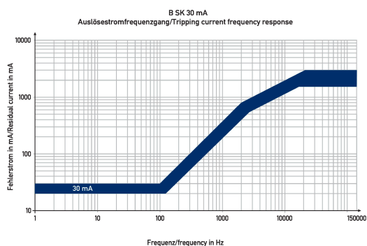
Diagramme Fehlerstromschutzschalter DFS 6 063-4/0,03-B SK NU
