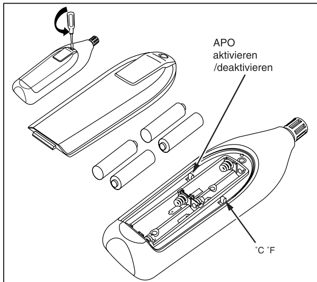
Abbildung 1. Batteriefach
