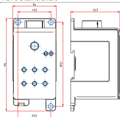
Montagehinweise | Assembly Details | Montage
