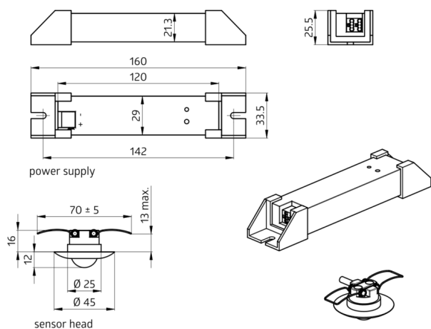
Bemaßung 93390
