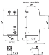
Maßbild DSH B TT 2P 255 FM
