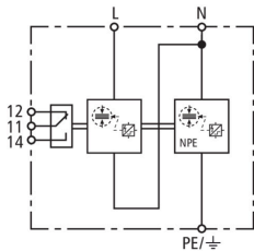
Prinzipialschaltbild DSH B TT 2P 255 FM
