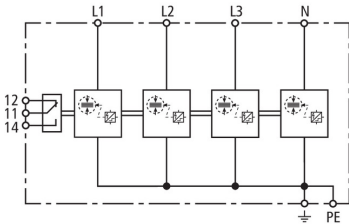
Prinzipschaltbild DSH TNS 255 FM
