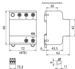
Maßbild DSH TNC 255 FM
