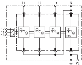
Prinzip Schaltbild DV M2 TT 255 FM
