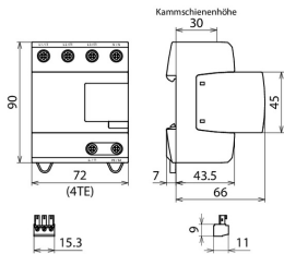
Maßbild DV M2 TT 255 FM
