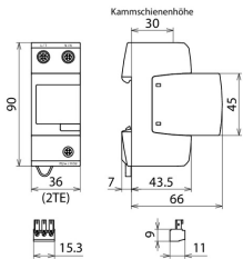
Maßbild DV M2 TT 2P 255 FM
