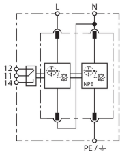
Prinzipialschaltbild DV M2 TT 2P 255 FM
