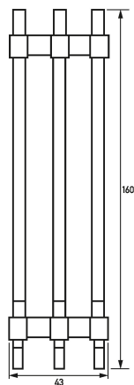
Maßzeichnung Gruppenansicht
