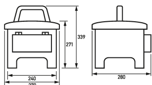
Maßzeichnung Gruppenansicht
