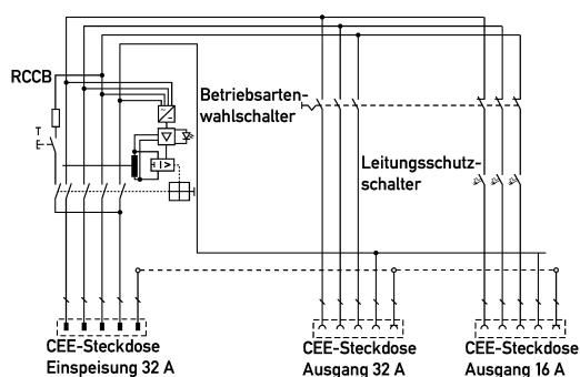
Anschlusschema
