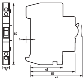
Maßzeichnung Gruppenansicht
