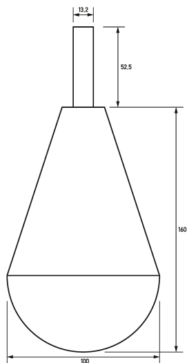
Maßzeichnung Gruppenansicht
