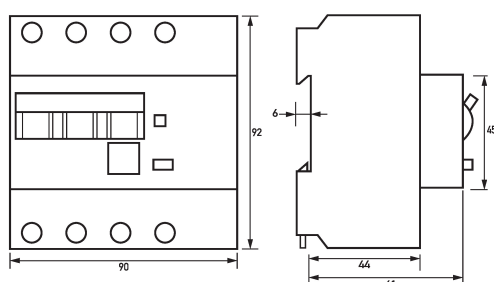
Maßzeichnung Gruppenansicht
