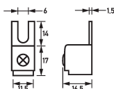
Maßzeichnung Gruppenansicht
