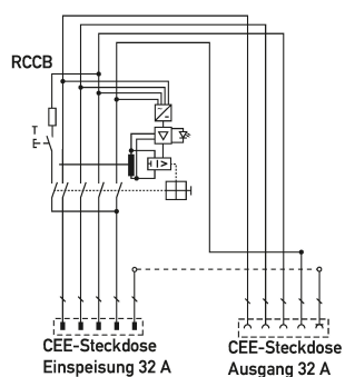
Anschlusschema
