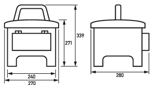
Maßzeichnung Gruppenansicht
