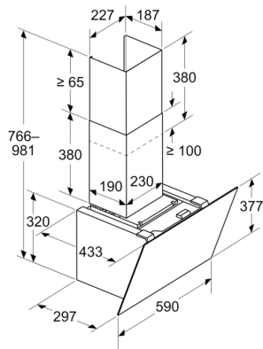
Maße in mm Gerät im Abluftbetrieb
