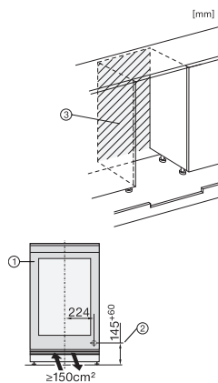
KWTUS7054F, KWTUS7055F, KWTUS7074F, KWTUS7096E, KWTUS7196E, Built-under, Installationsskizze (*Fußnote) (Skizze)
