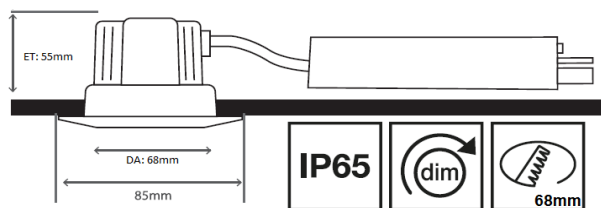
Ansicht 2
