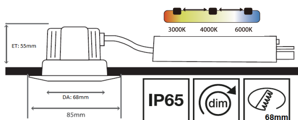
Ansicht 2
