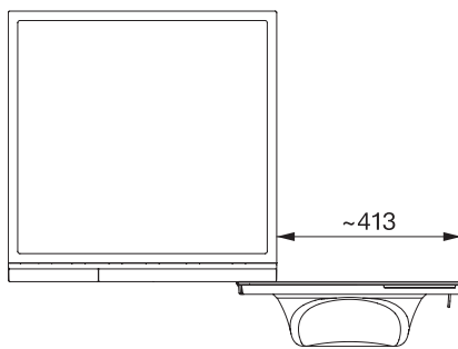
W2 mit Glastür, 17 Grad Blende, Maße in mm
