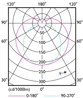
LEDtube MAS 36W G5 5200lm
