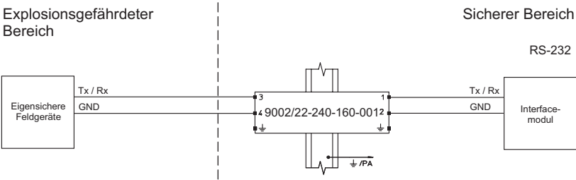
Anwendungsfall mit RS 232
