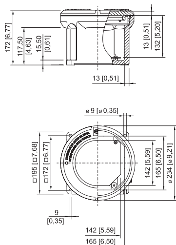
Gehäuse Größe 3 ohne Schauglas
