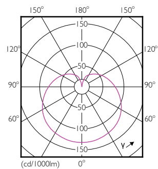
CorePro LEDlustre 4-25W E14 827 FR P45
