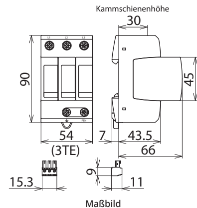
Maßbild
