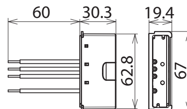
Maßbild
