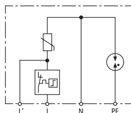
Prinzipschaltbild
