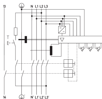
Anschlusschema
