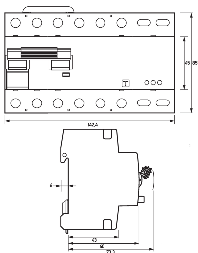
Maßzeichnung Gruppenansicht
