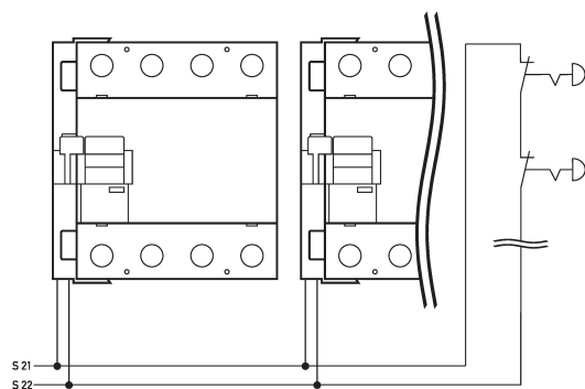
Anschlusschema
