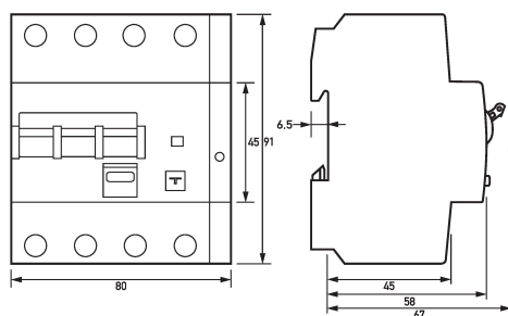
Maßzeichnung Gruppenansicht
